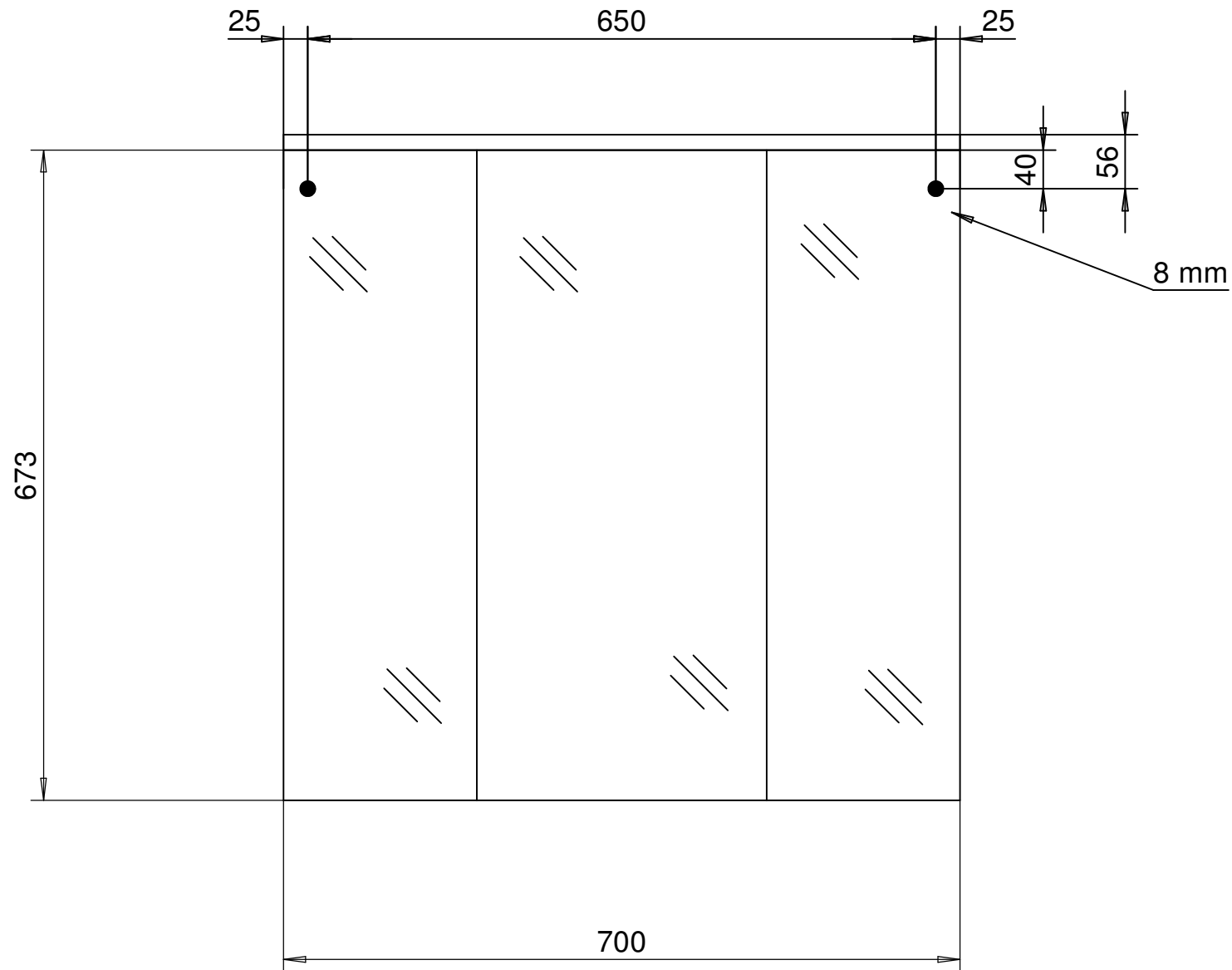
Montagemaße Next SP 70
