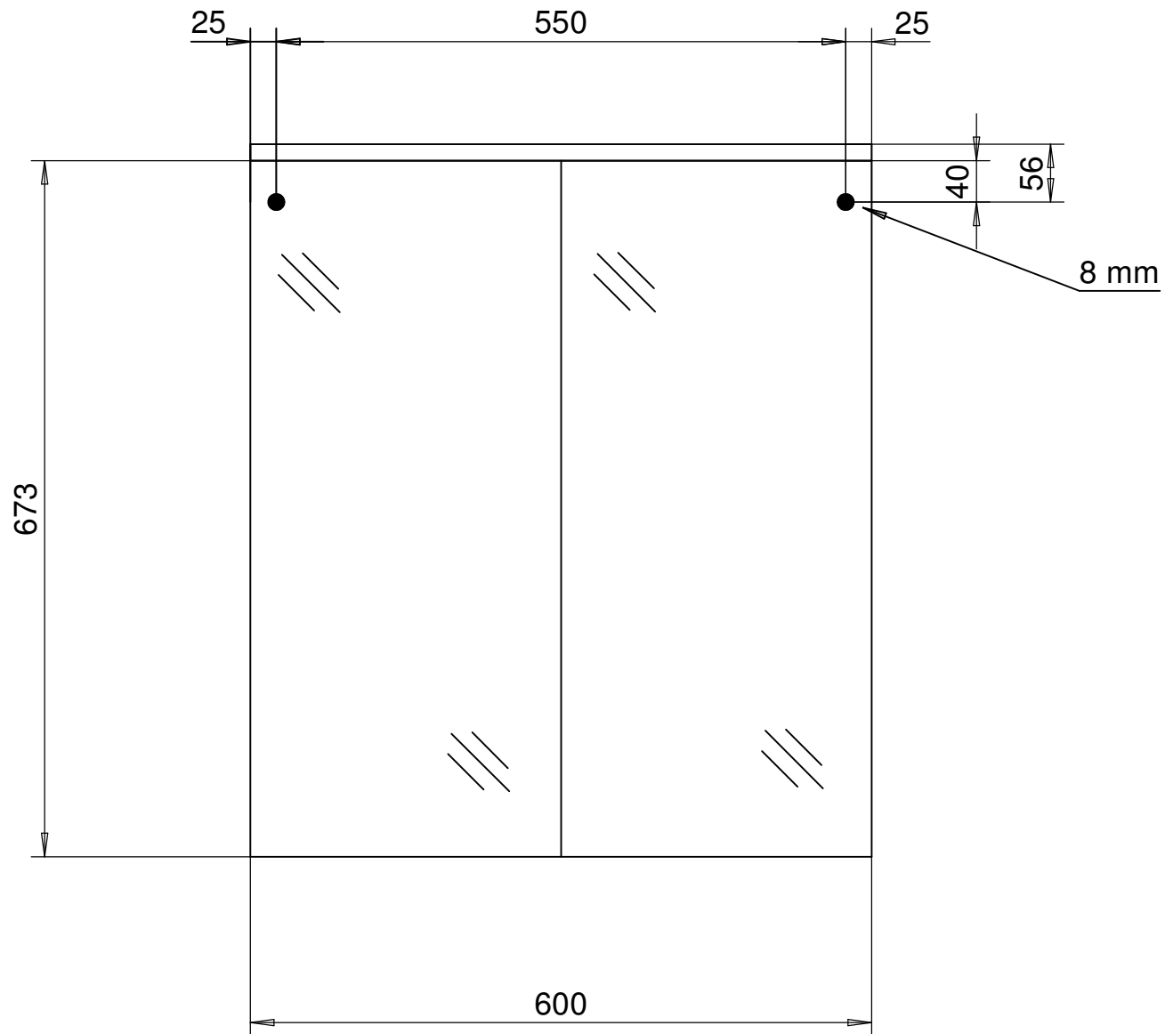
Montagemaße Next SP 60
