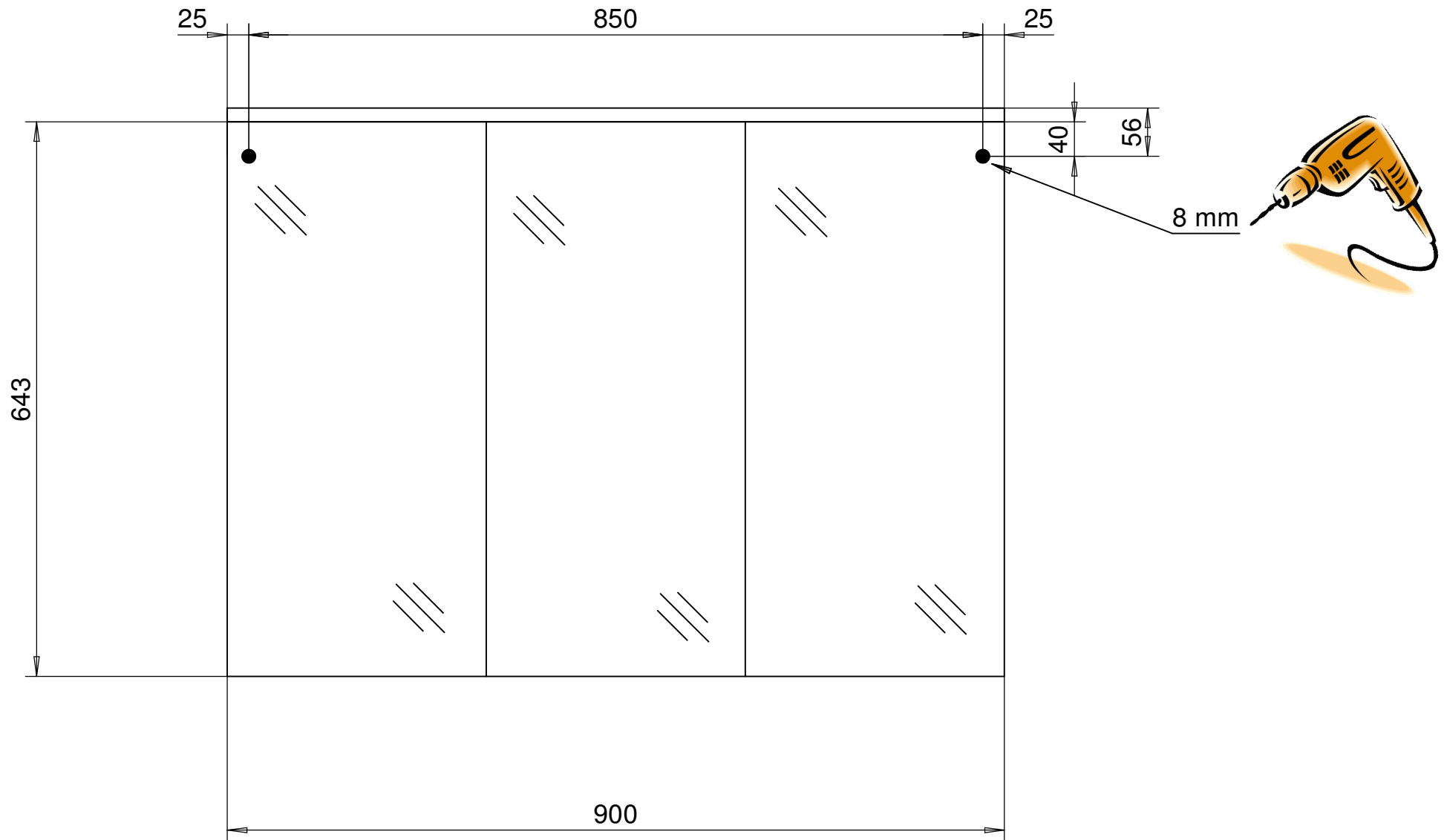
Montagemaße Multi SP 90
