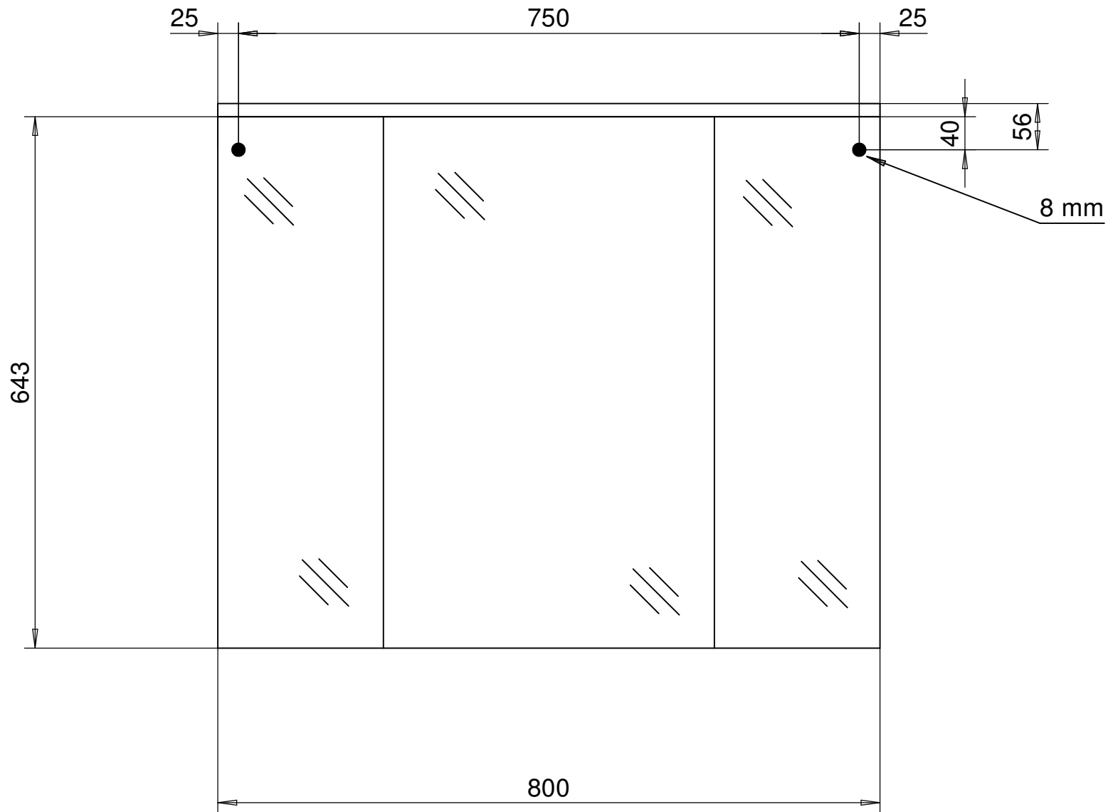
Montagemaße Multi SP 80
