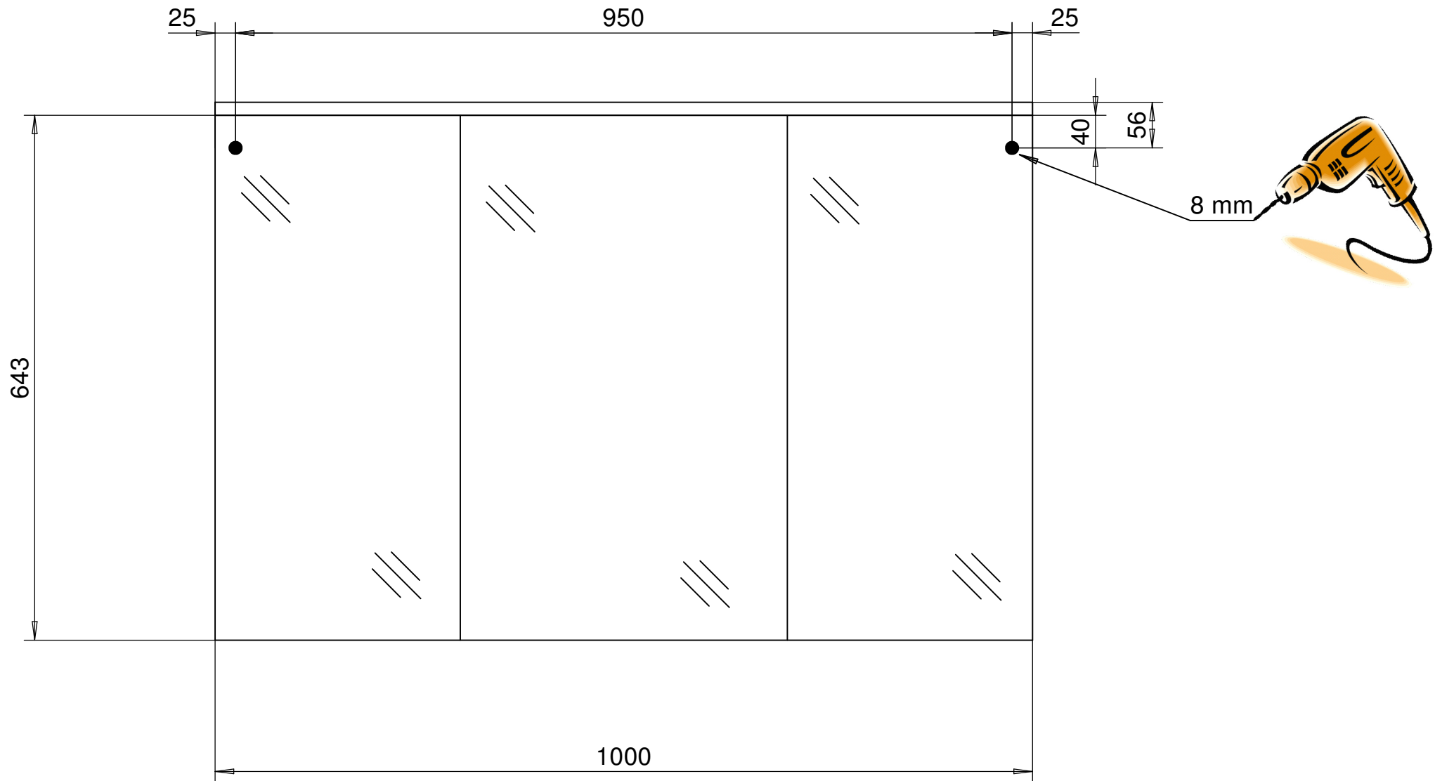
Montagemaße Multi SP 100
