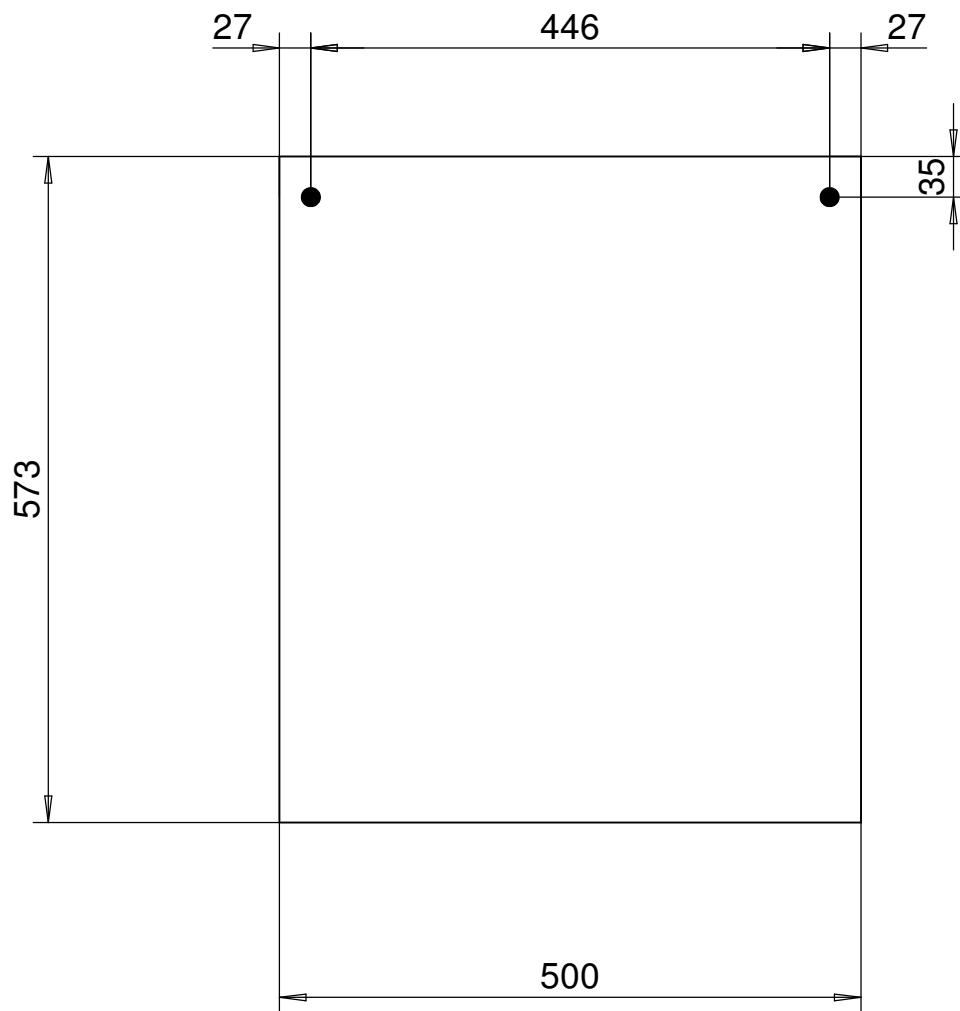
Montagemaße Küche H 50
